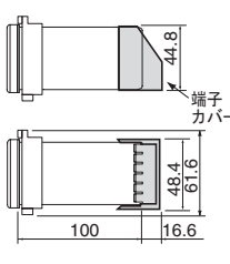
CB100用端子カバー 型式: KCA100-517
