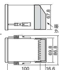
CB700用端子カバー 型式: KCA700-53
