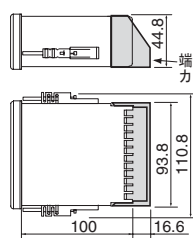
CB500/400用端子カバー 型式: KCA400-513
