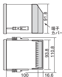
CB900用端子カバー 型式: KCA900-58
