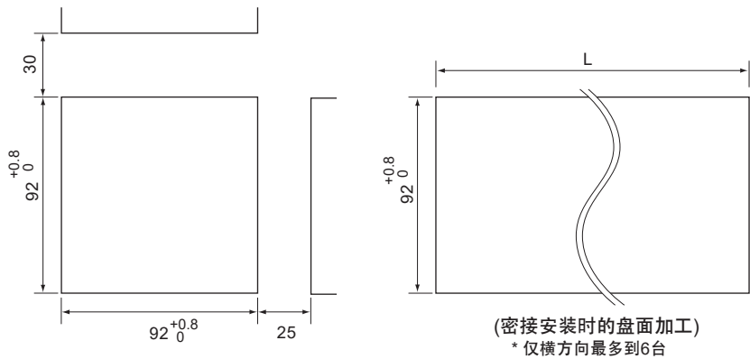
盘面加工
