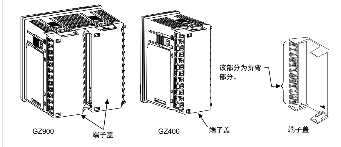
图 3.4 关于端子盖的安装参考图与折弯部分
