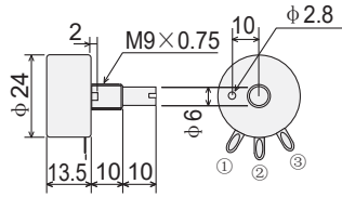
电位器 (电阻值5kΩ, 变化特性:B)
