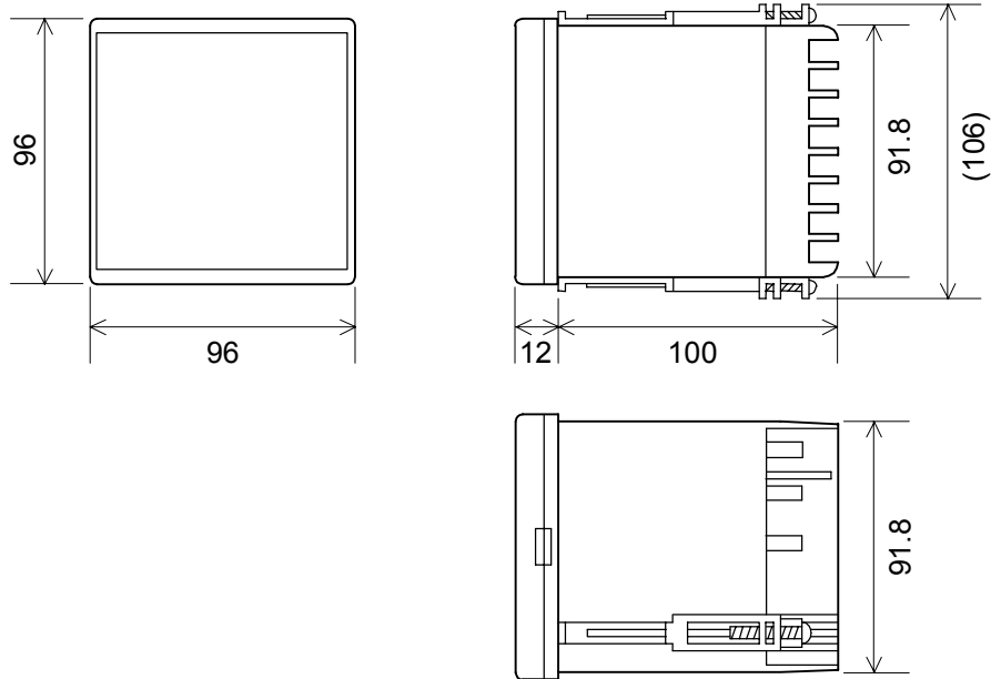
Fig. 2.1 Dimensions
