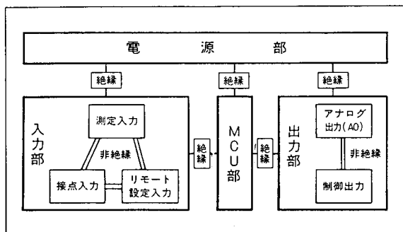
回路構成
