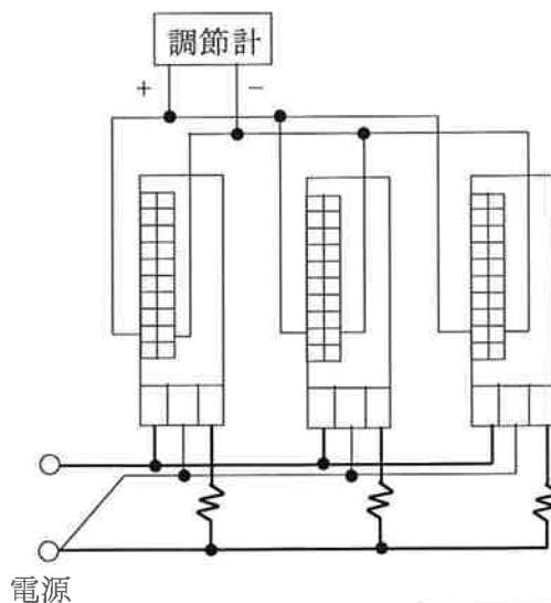
DC0 ~ 5V / DC1 ~ 5V 入力タイプ (パラレル接続)
