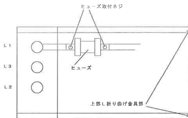
図3 ヒューズ取付ネジの位置図 (上から見た図)
