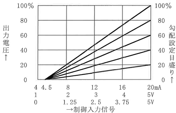
勾配出力特性図
