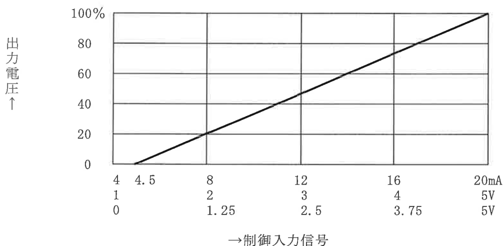
比例制御入出力特性図
