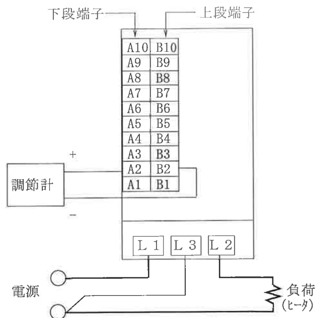
DC0 ~ 5V / DC1 ~ 5V 入力タイプ (パラレル接続)
