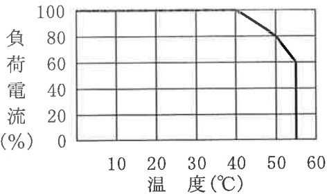
負荷電流温度特性
