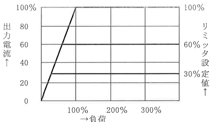
電流リミッタ特性図
