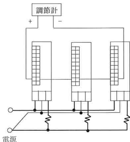
DC4 ~ 20mA 入力タイプ (シリーズ接続)
