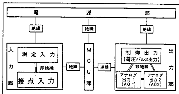
REX-F9メモリエリア回路構成例
