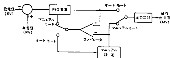
オート/マニュアル切替時の バランスレスバンプレスの概念図
