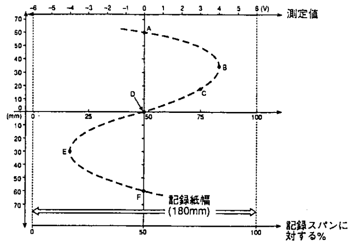
図8.2 通常記録例
