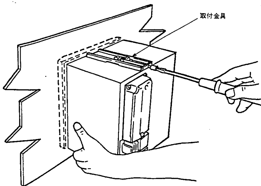
図3.1 取付方法
