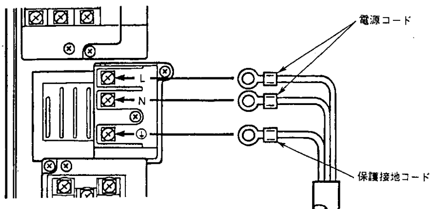
図3.4 電源の配線
