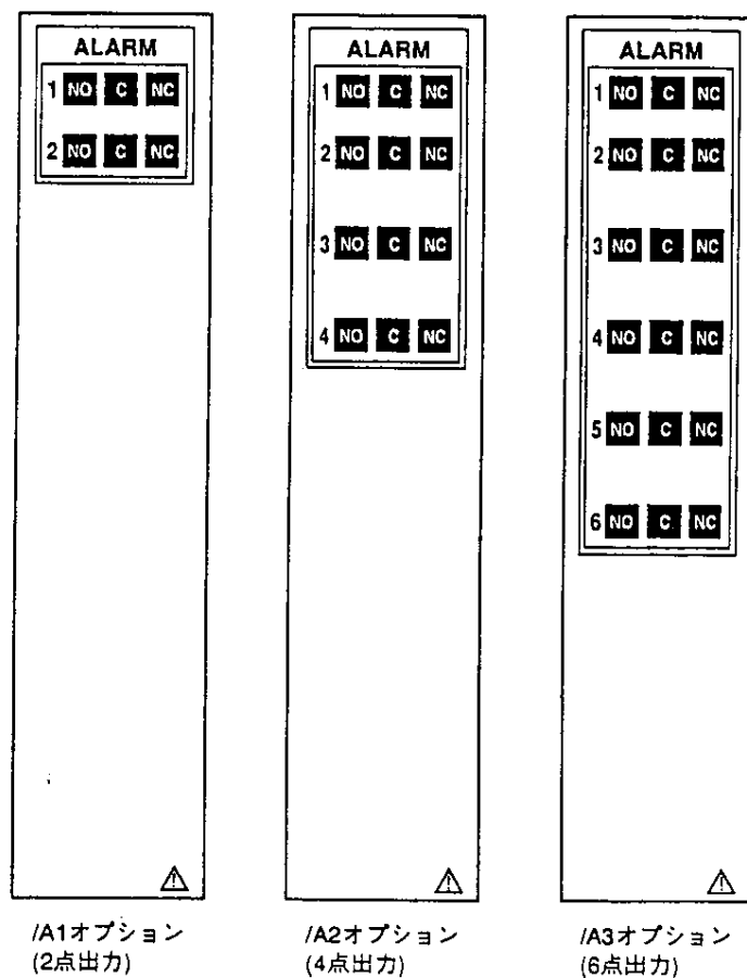
図3.9 警報出力端子
