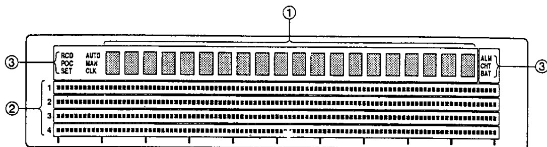
図4.3 ディスプレイのレイアウト(4ペンモデル)
