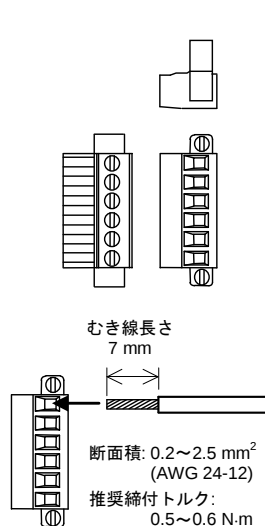
[SRVP-02] サイドネジタイプ
