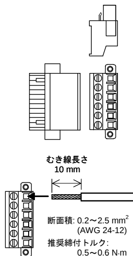
[SRVP-01] フロントネジタイプ
