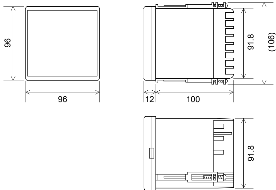
Fig. 2.1 Dimensions
