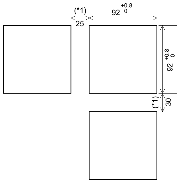
Fig. 2.1 Dimensions
