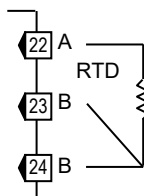
RTD input
