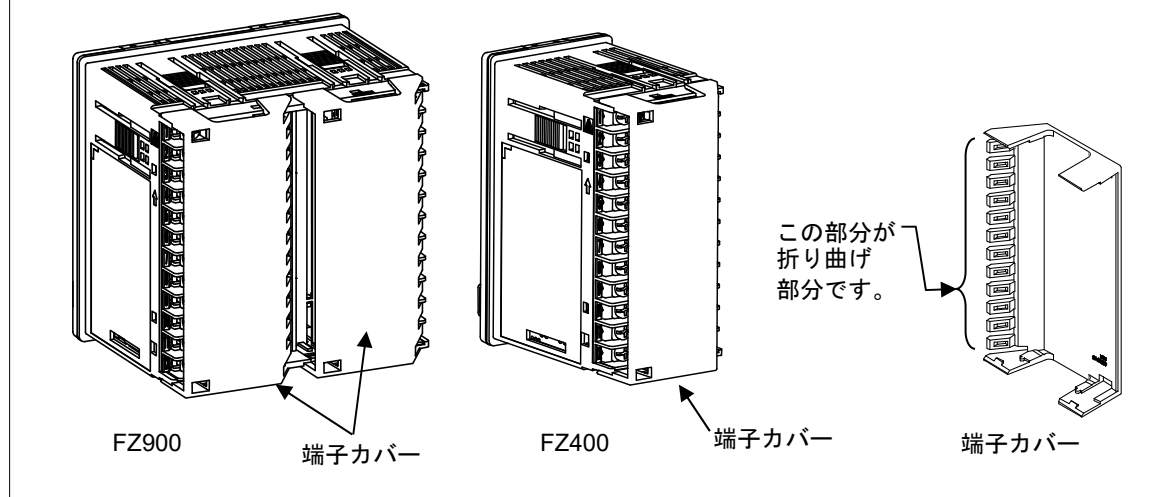
図 3.4 端子カバーの装着イメージと折り曲げ部分について (FZ400/FZ900 の場合のみ)
